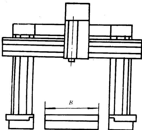
图 3 龙门架和横梁移动式
