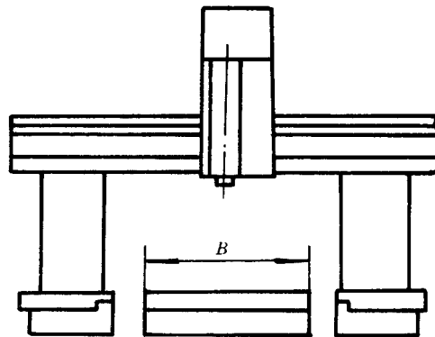
图 4 龙门架移动横梁固定式
