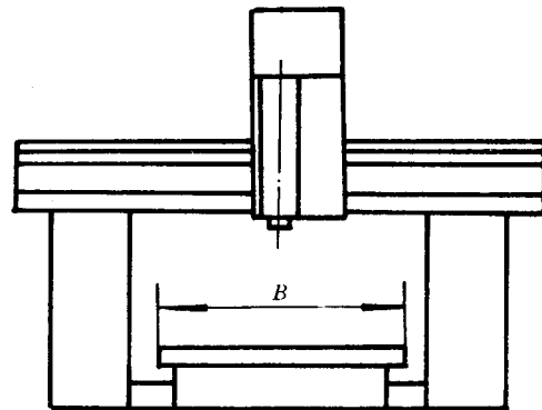
图 2 工作台移动横梁固定式
